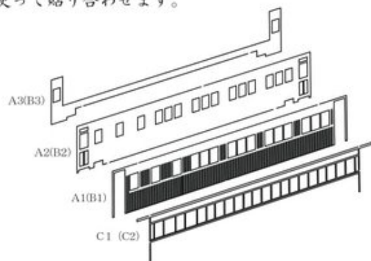
側板
